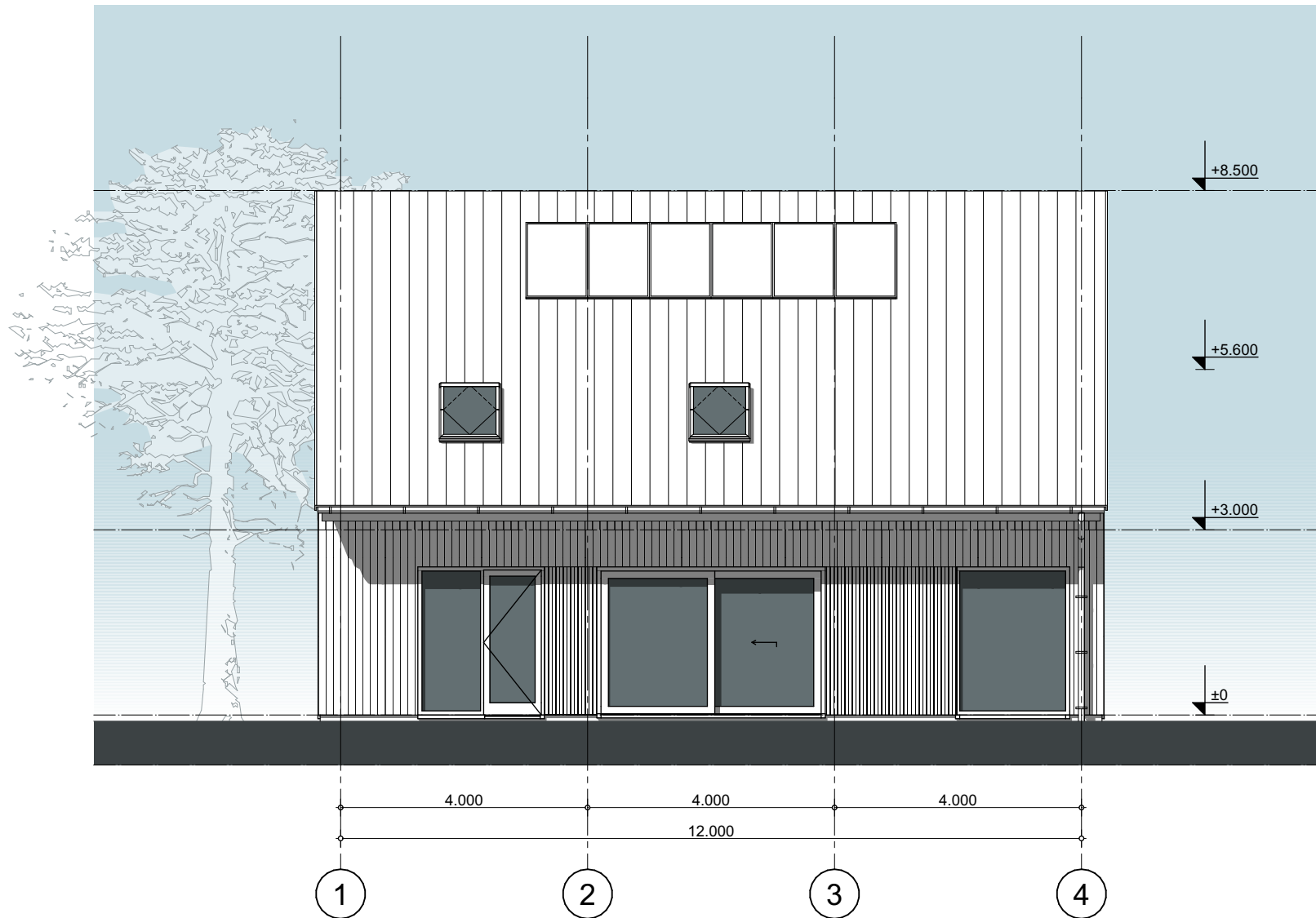
Achteraanzicht
