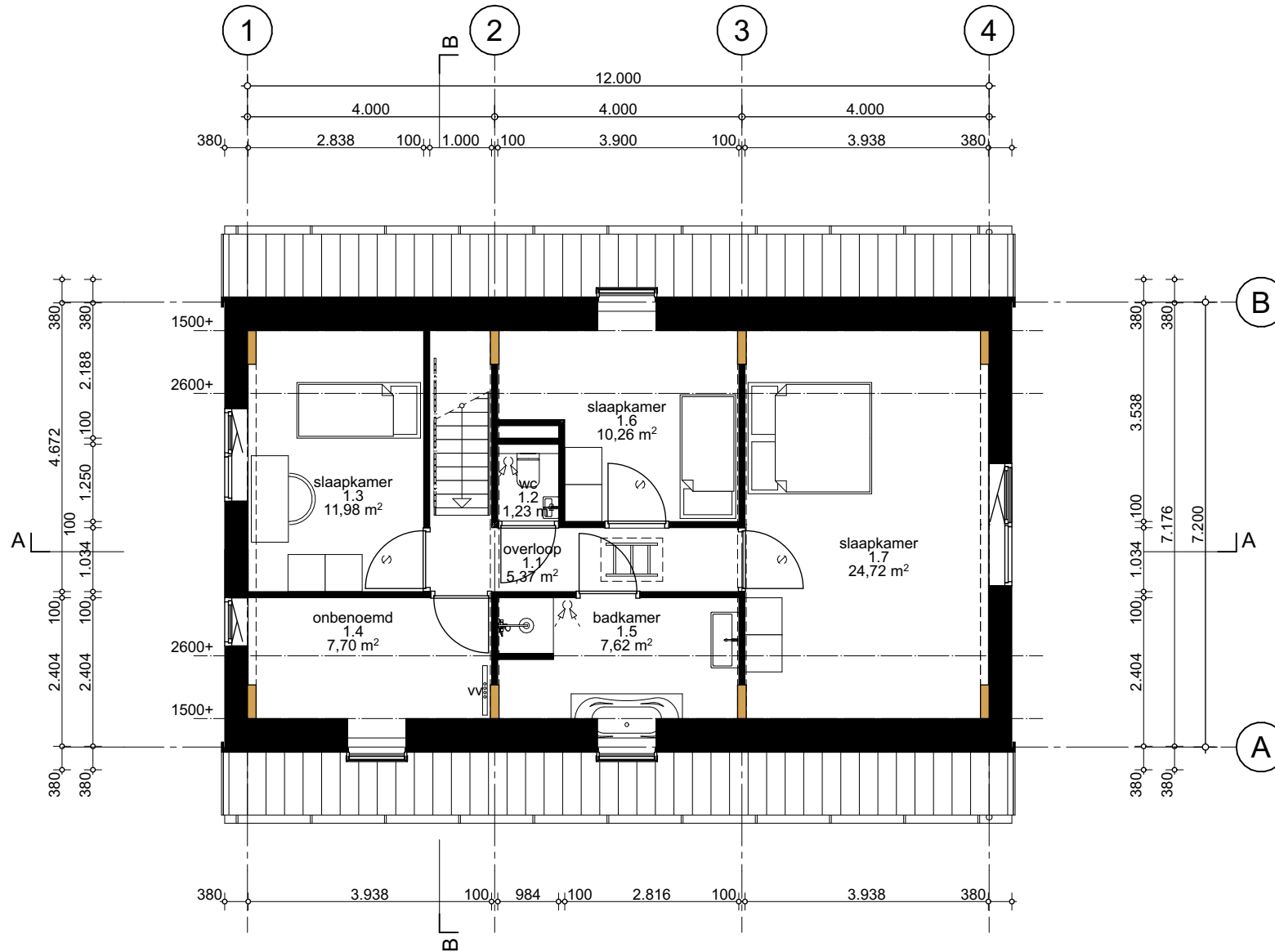
1e verdieping (3.000+P)
