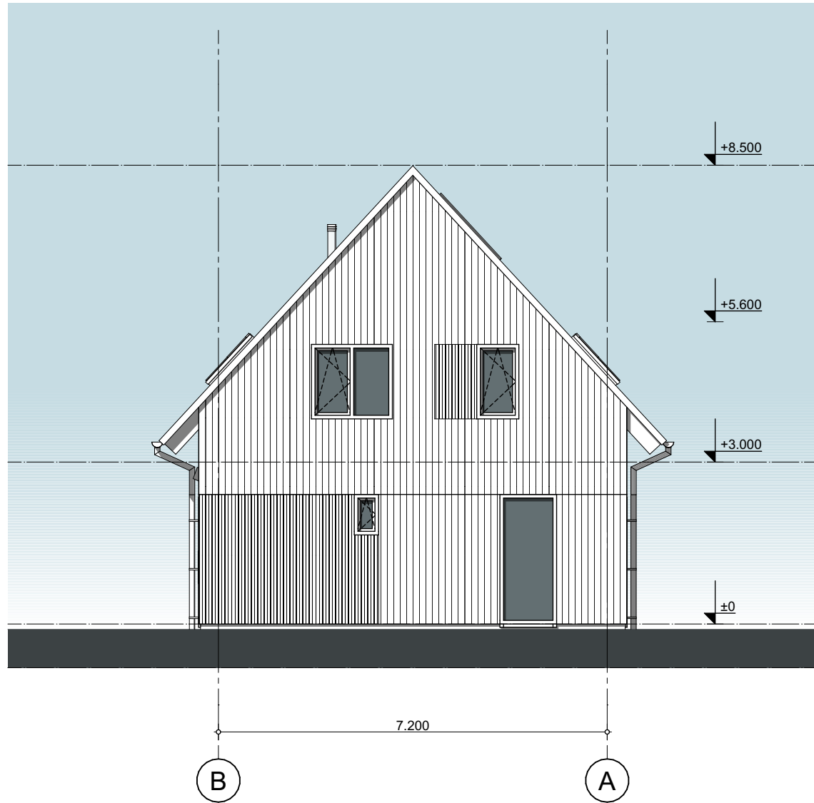
Rechter zijaanzicht
