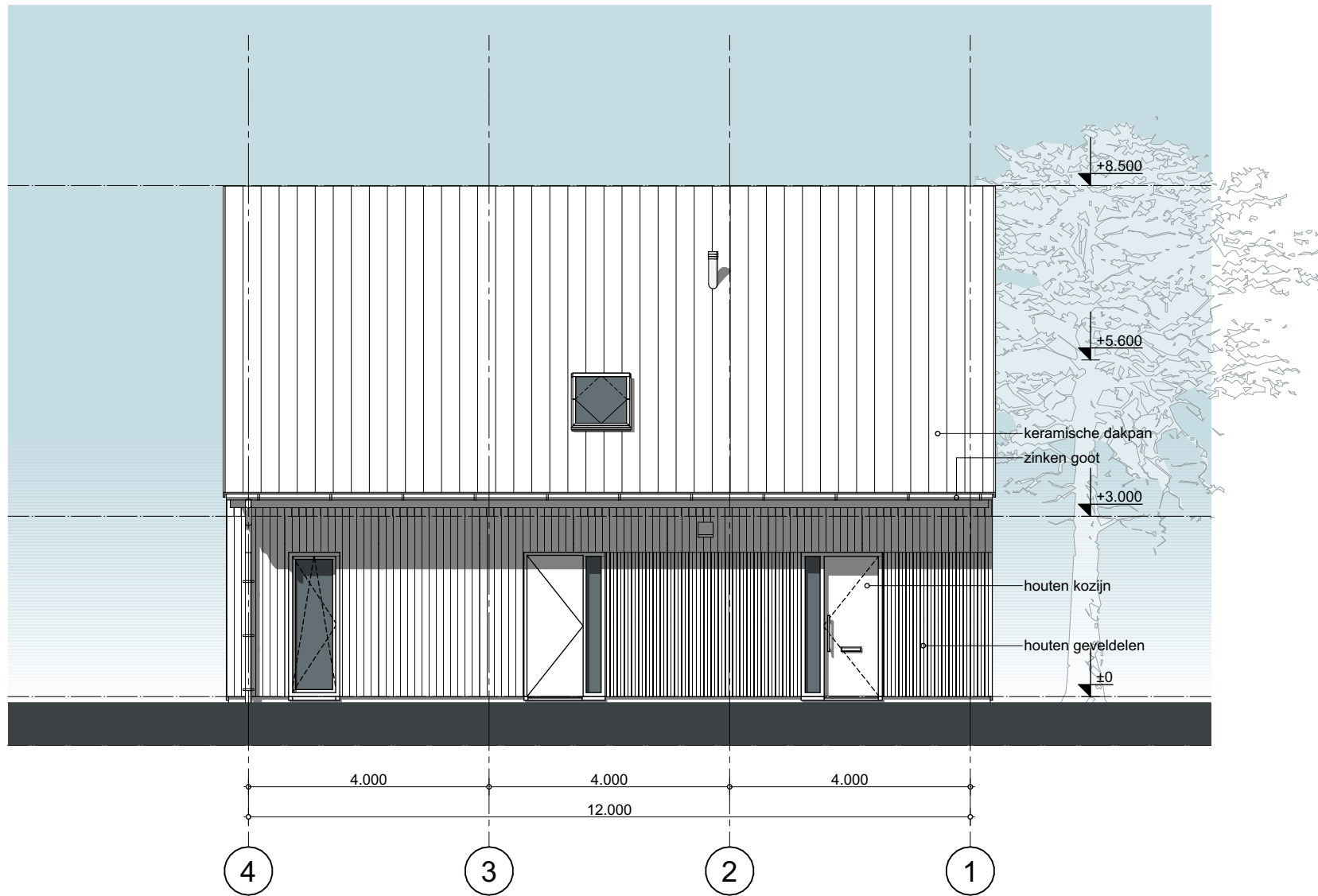
Voorraanzicht
