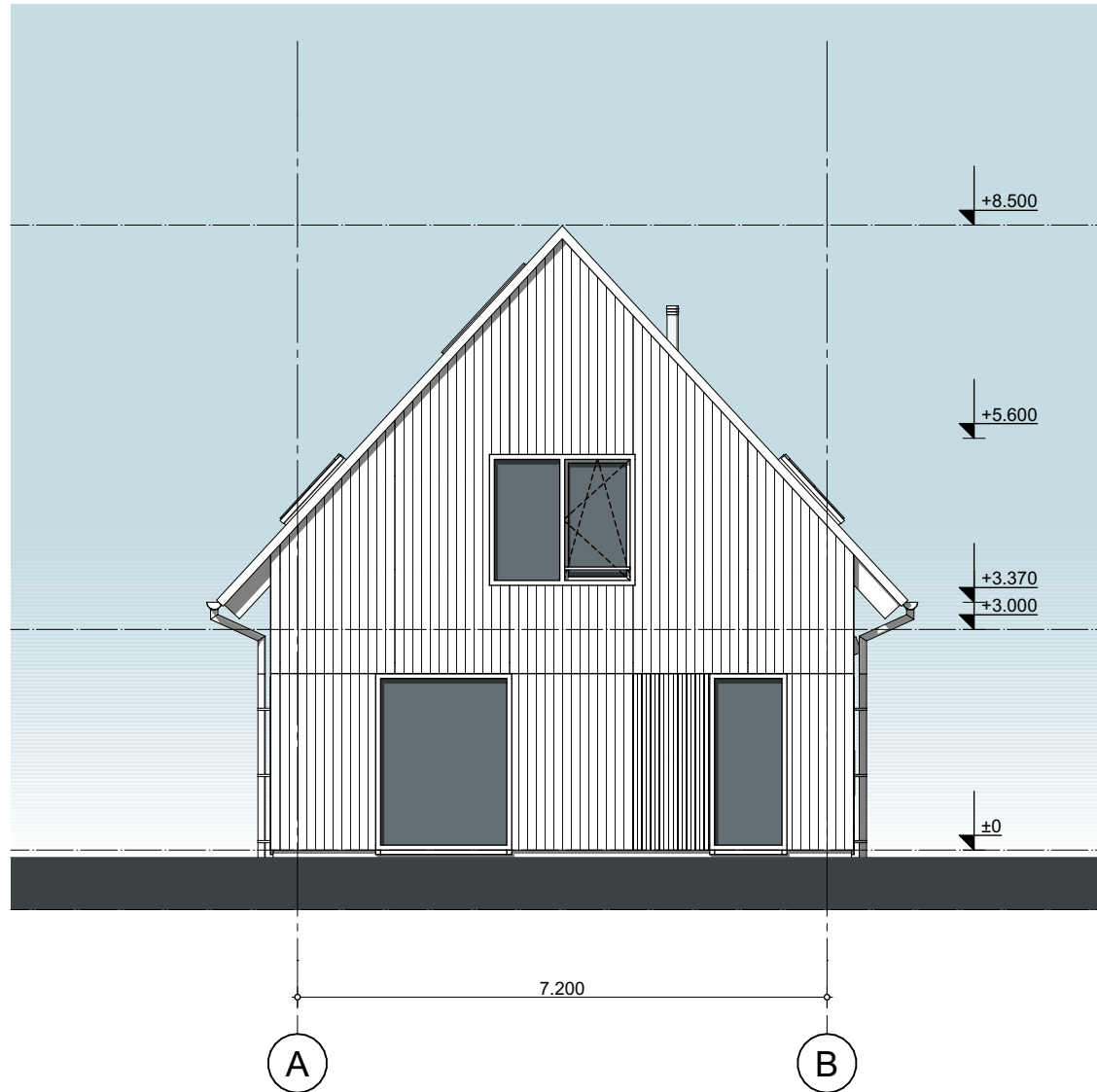
Linker zijaanzicht
