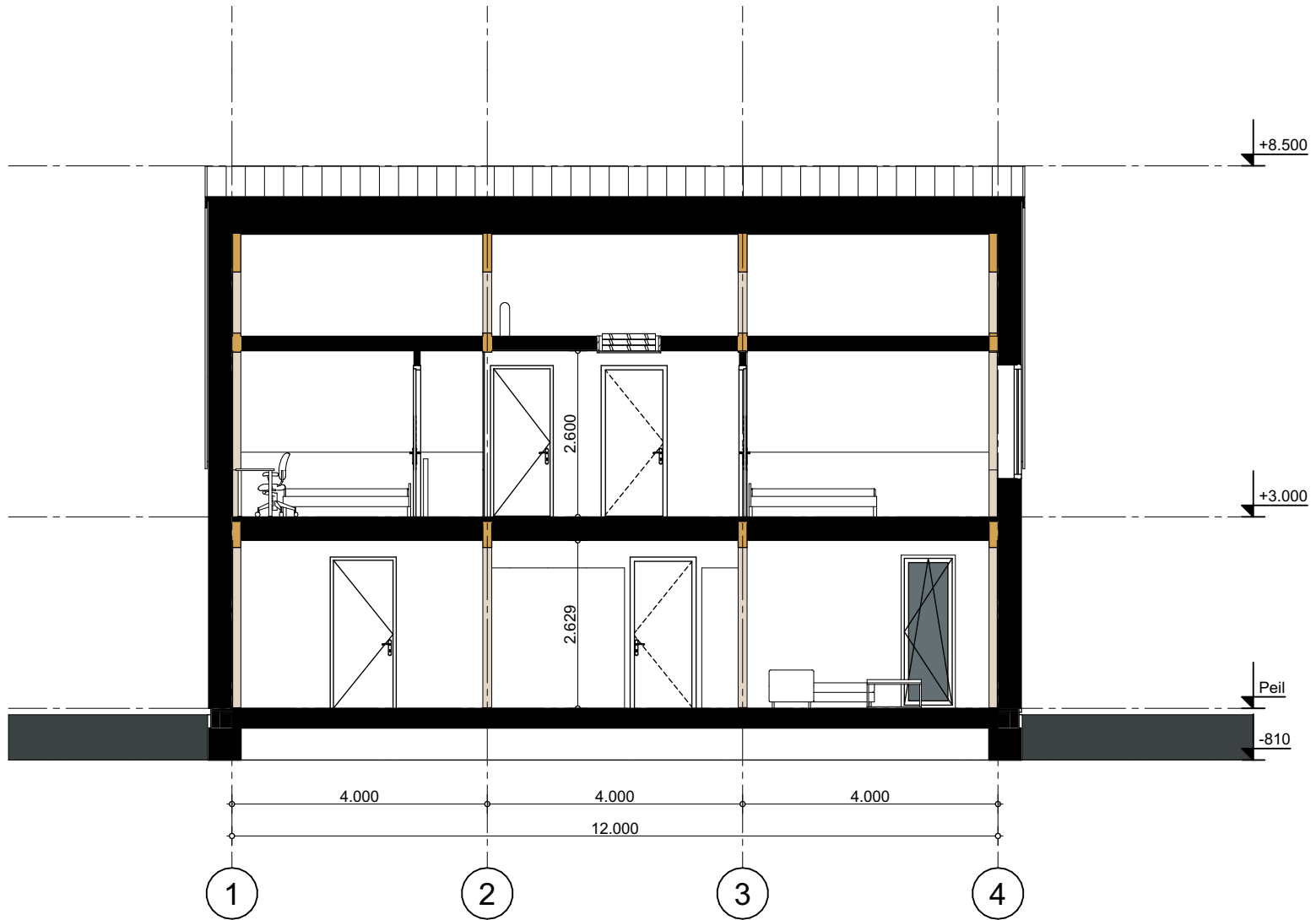
Doorsnede A-A
