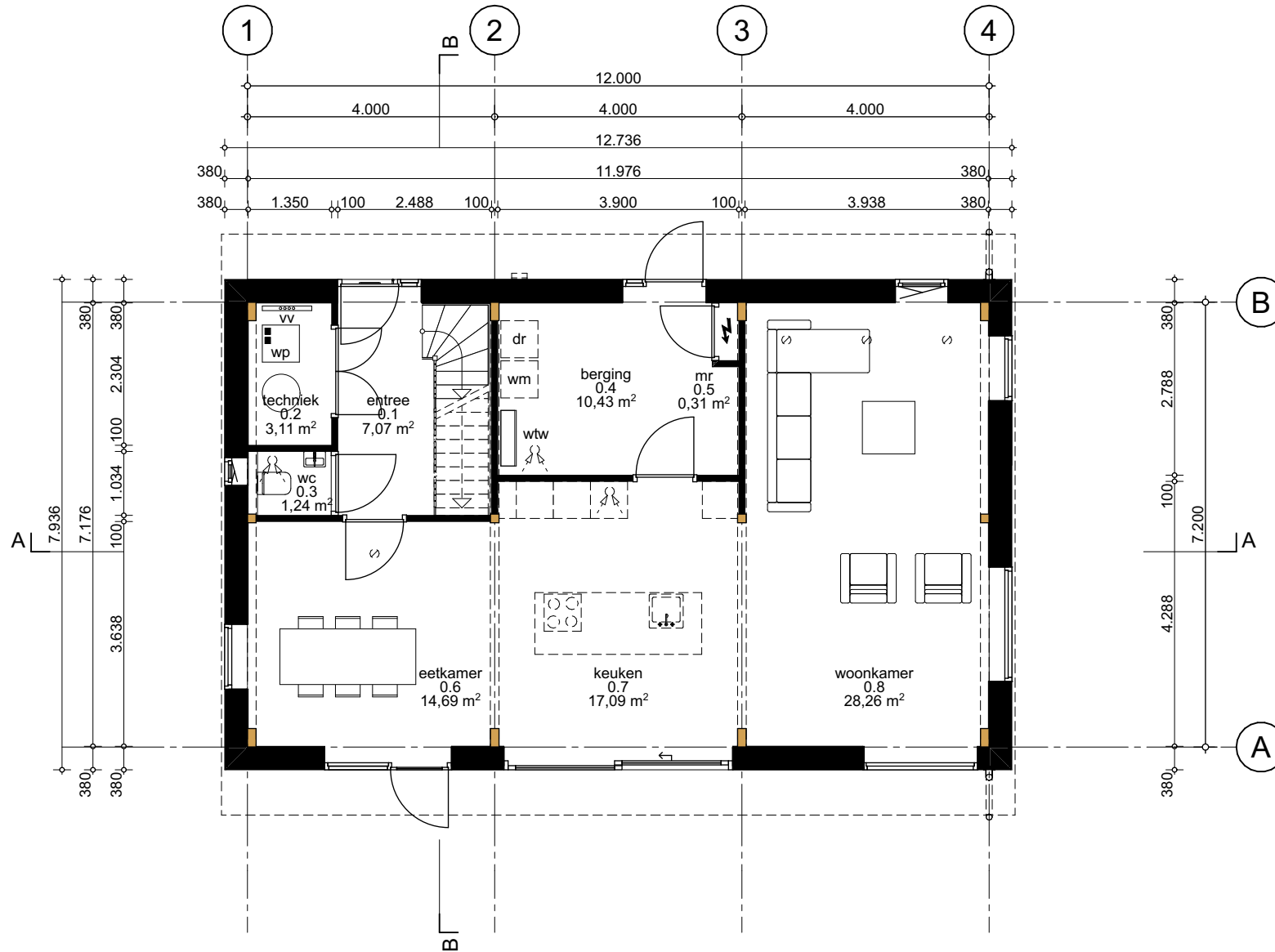
Begane grond (PEIL=0)
