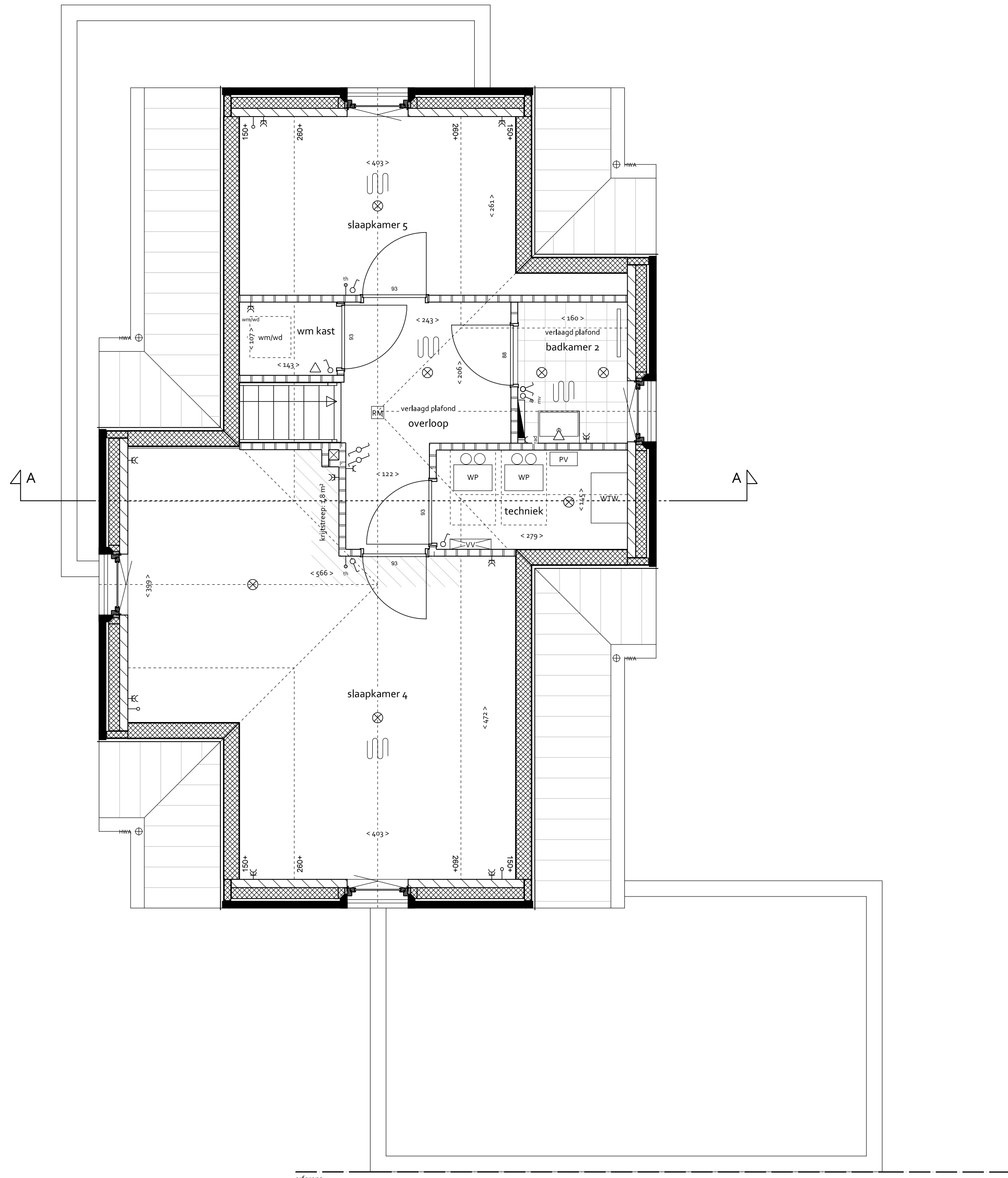
TWEDE VERDIEPING 1:50
