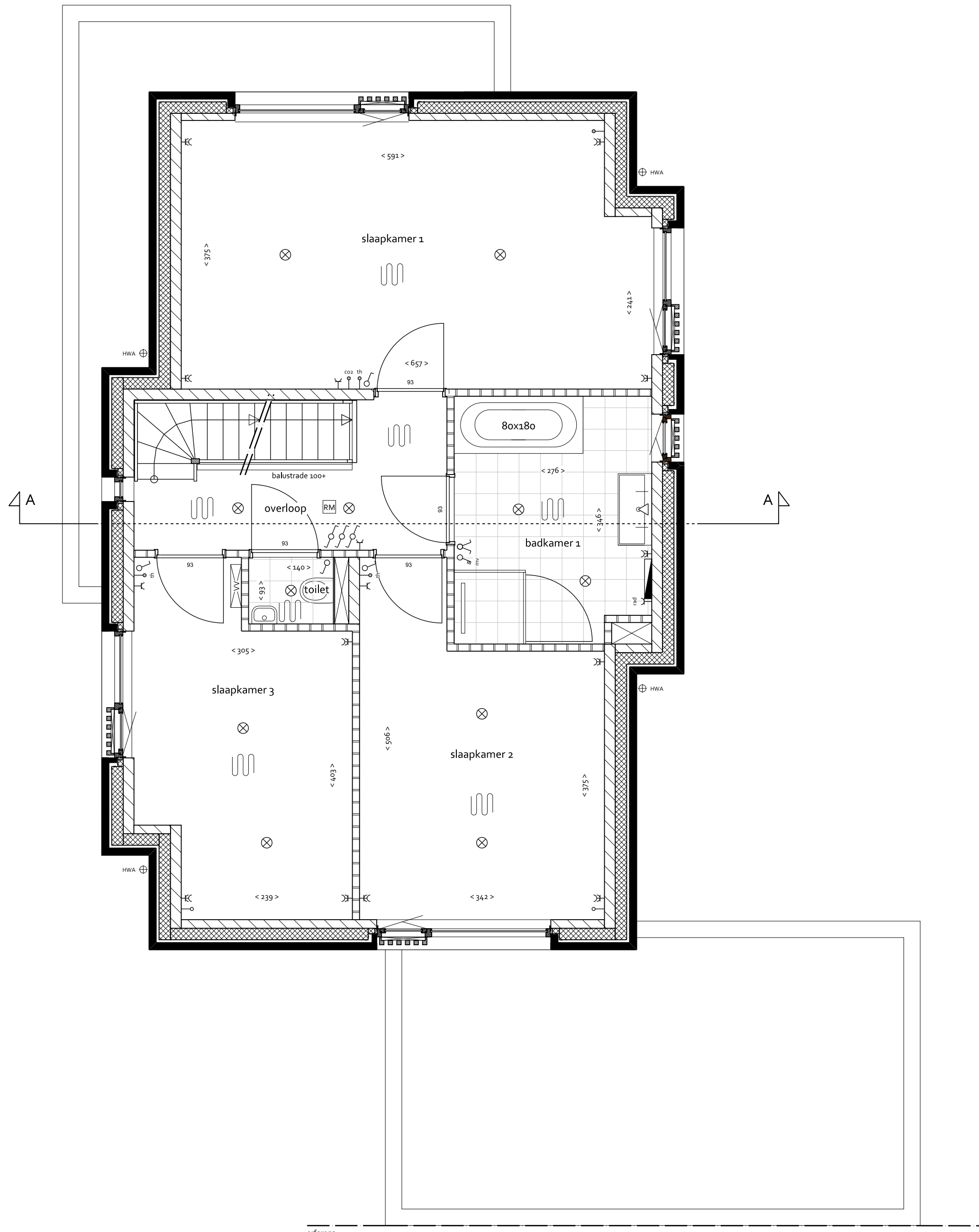
EERSTE VERDIEPING 1:50
