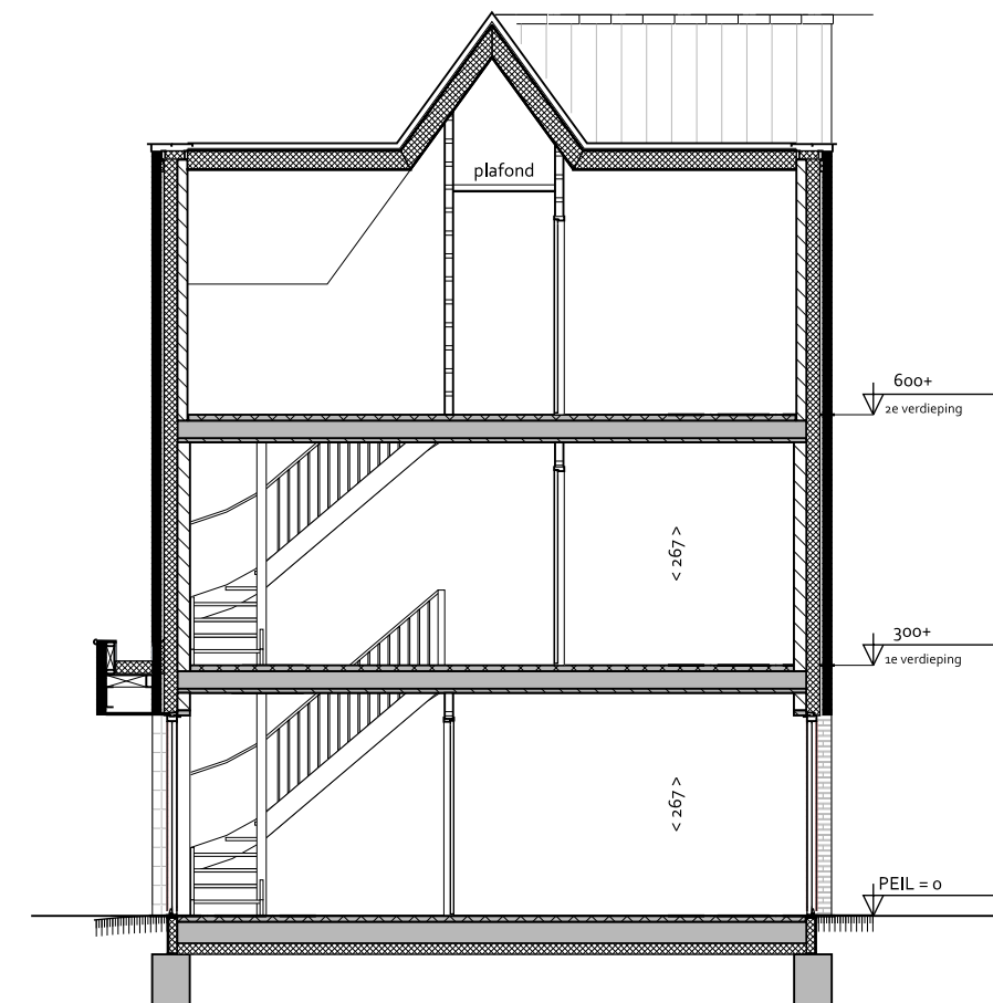
DOORSNEDE A-A 1:100
