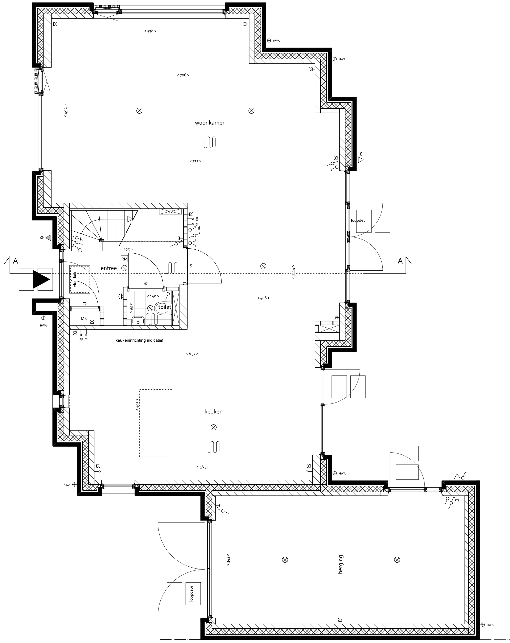
BEGANE GROND 1:50
