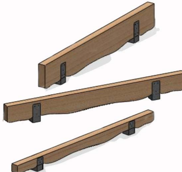
balken voor op de helling
