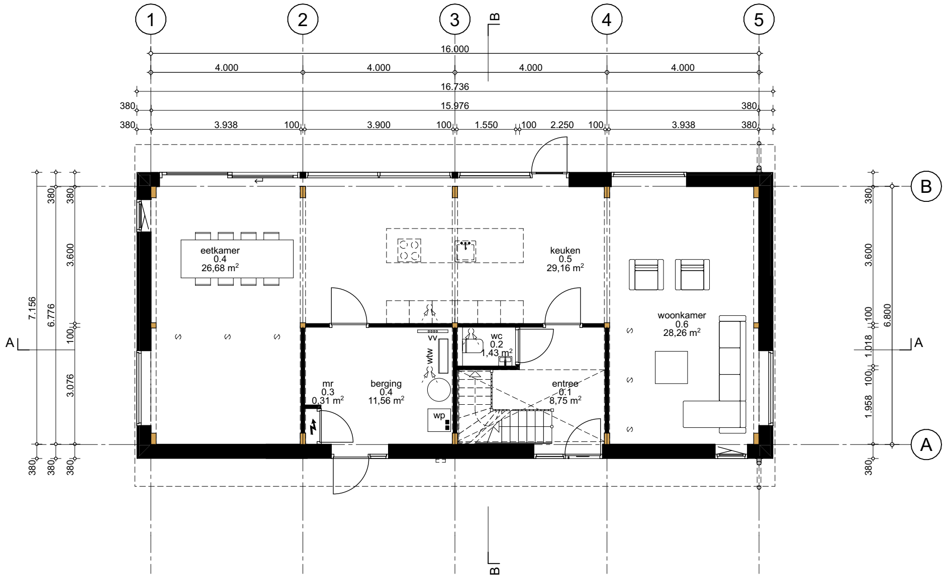
Begane grond (PEIL=0)
