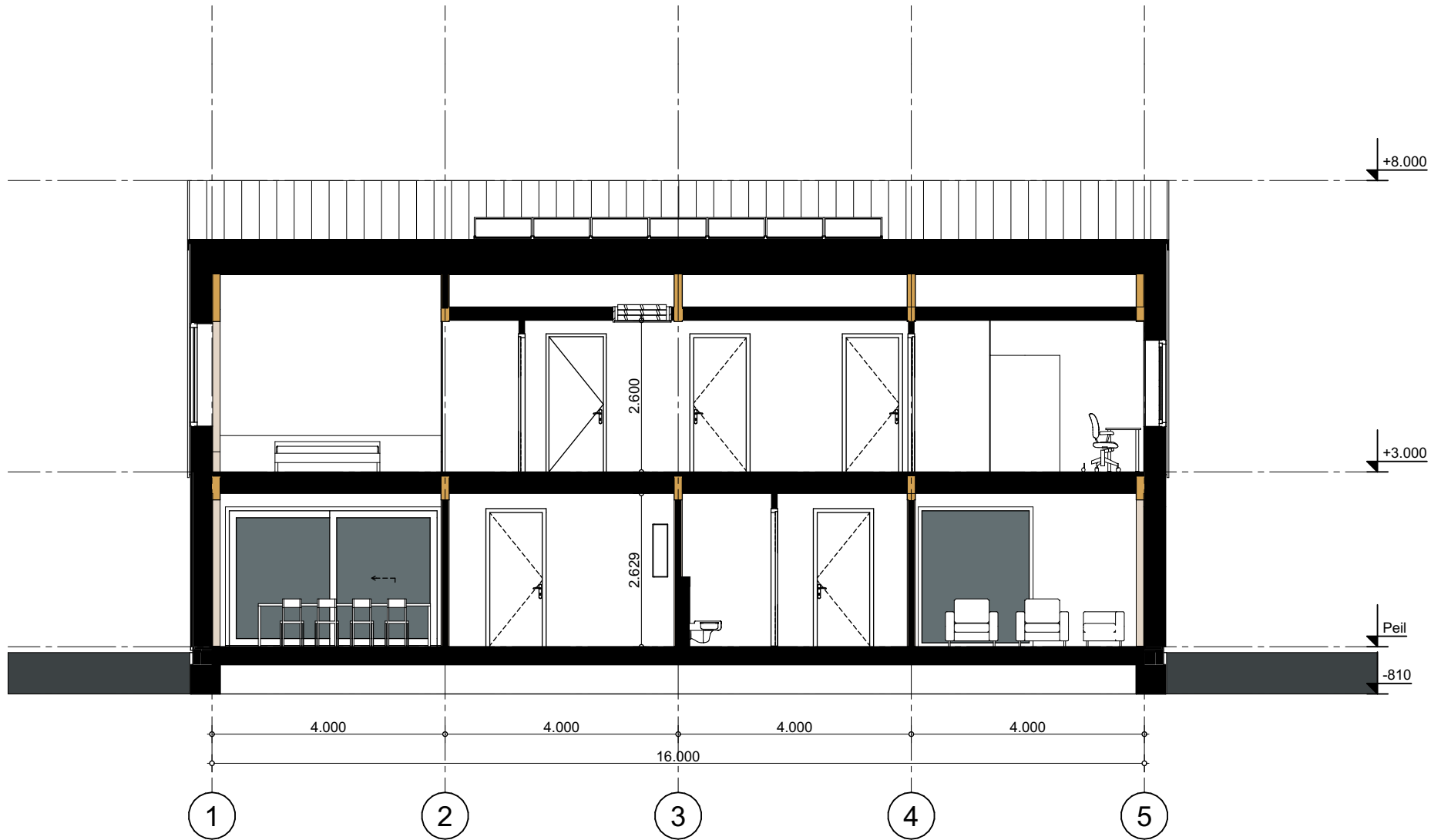
Doorsnede A-A
