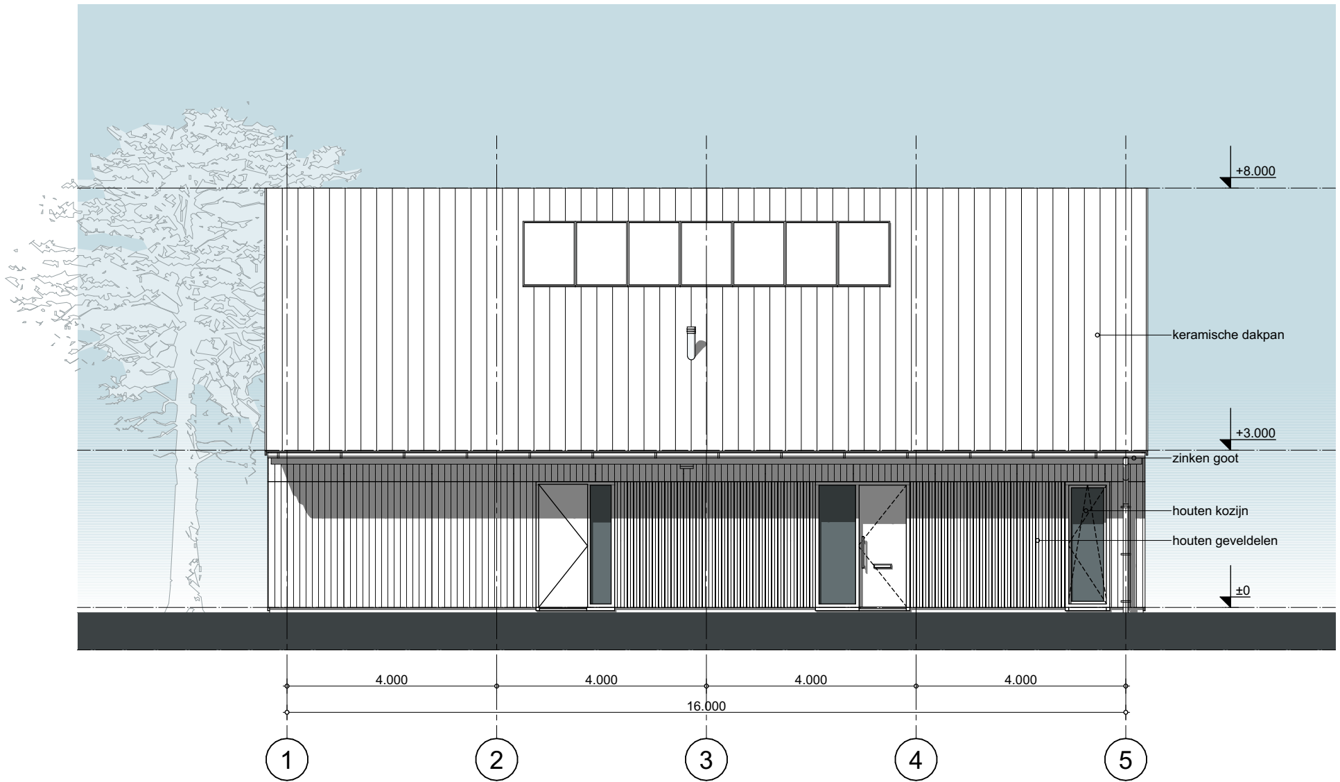
Vooranzicht
