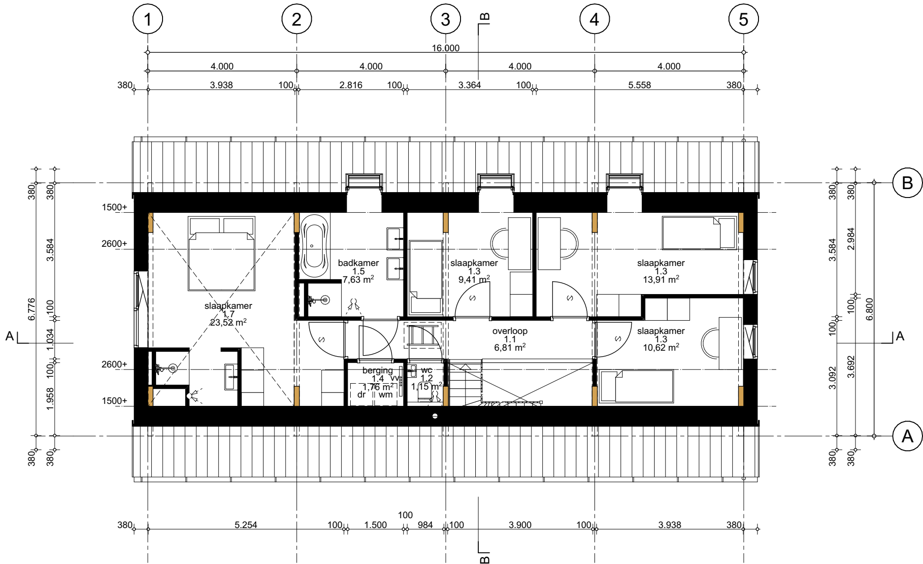
1e verdieping (3.000+P)
