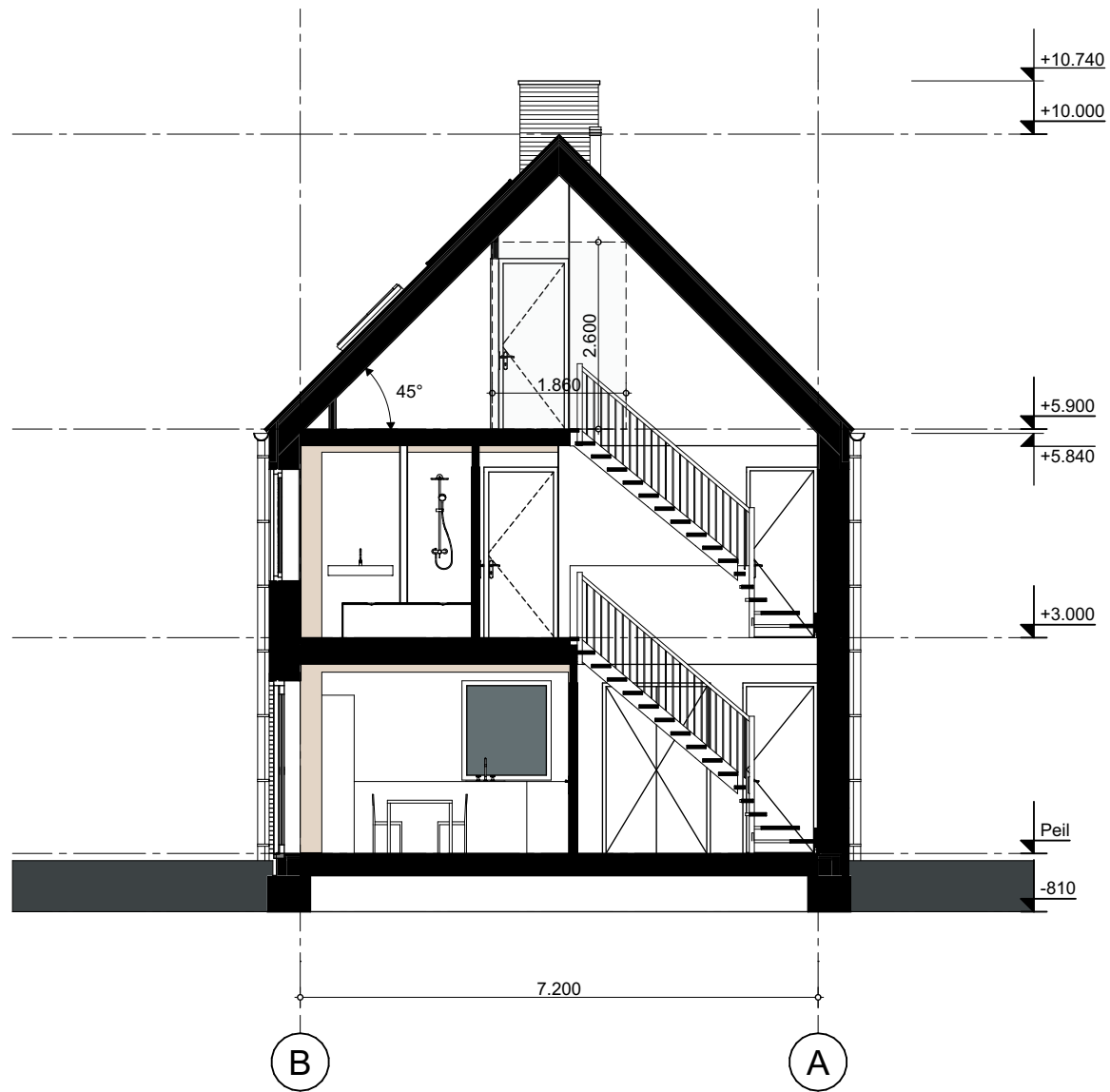
Doorsnede B-B
