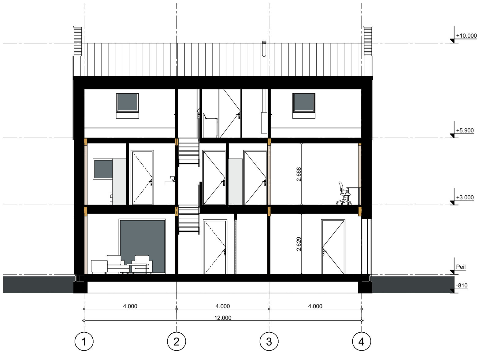
Doorsnede A-A
