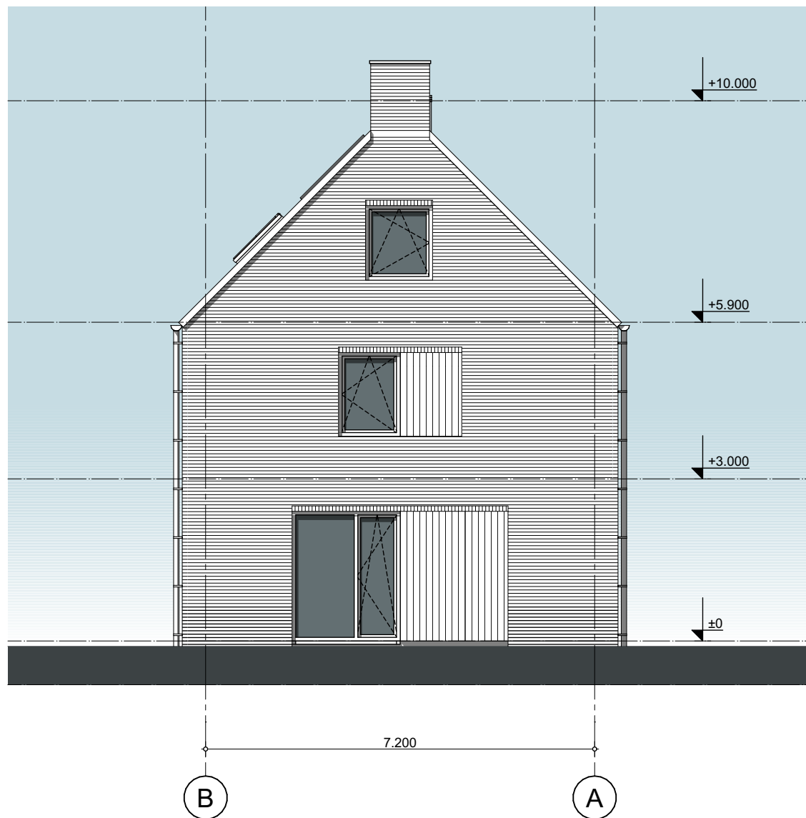
Linker zijaanzicht
