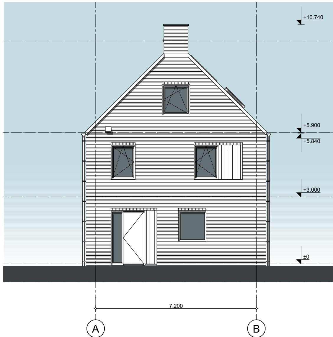
Rechter zijaanzicht
