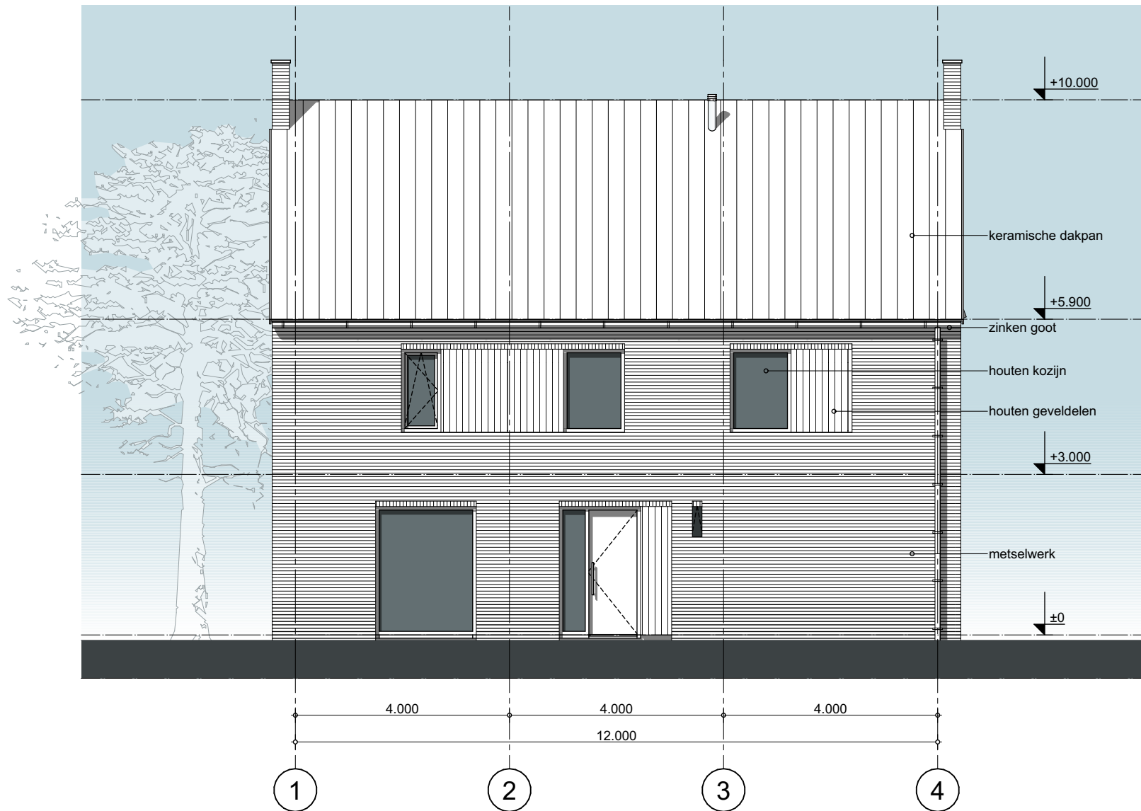
Voorraanzicht
