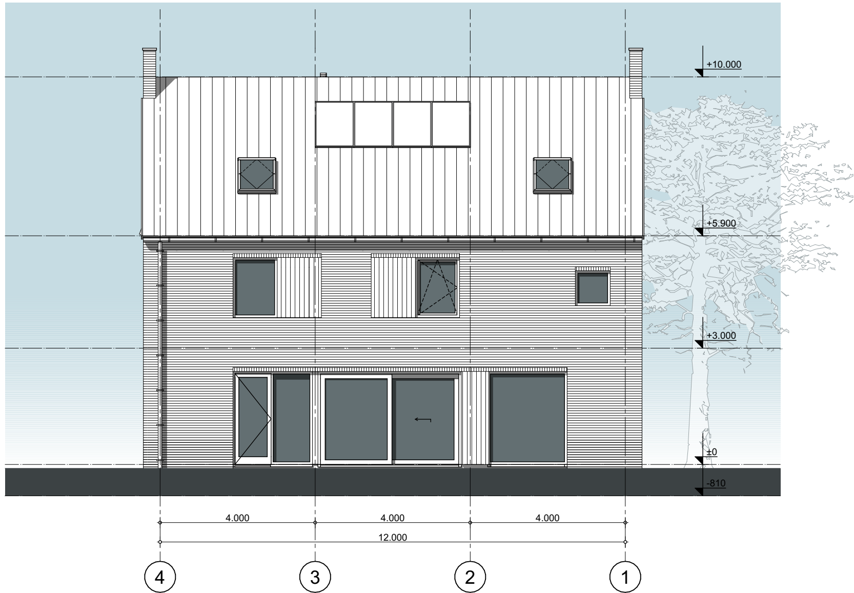
Achteraanzicht
